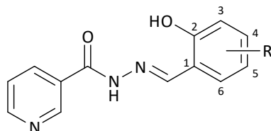
Slika 1: Strukture aromatskih hidrazona: R = H ( 1 ); 3-OCH 3 ( 2 ); 4-OCH 3 ( 3 ); 5-OCH 3 ( 4 ).
