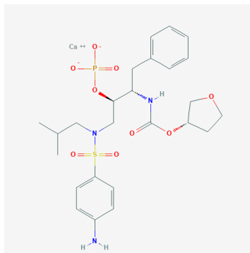
Slika 1: Molekula fosamprenavir-kalcija.
