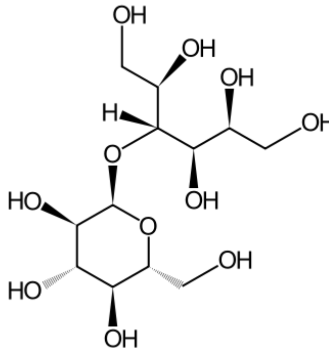
4-O-α-glukopiranozil-D-sorbitol
