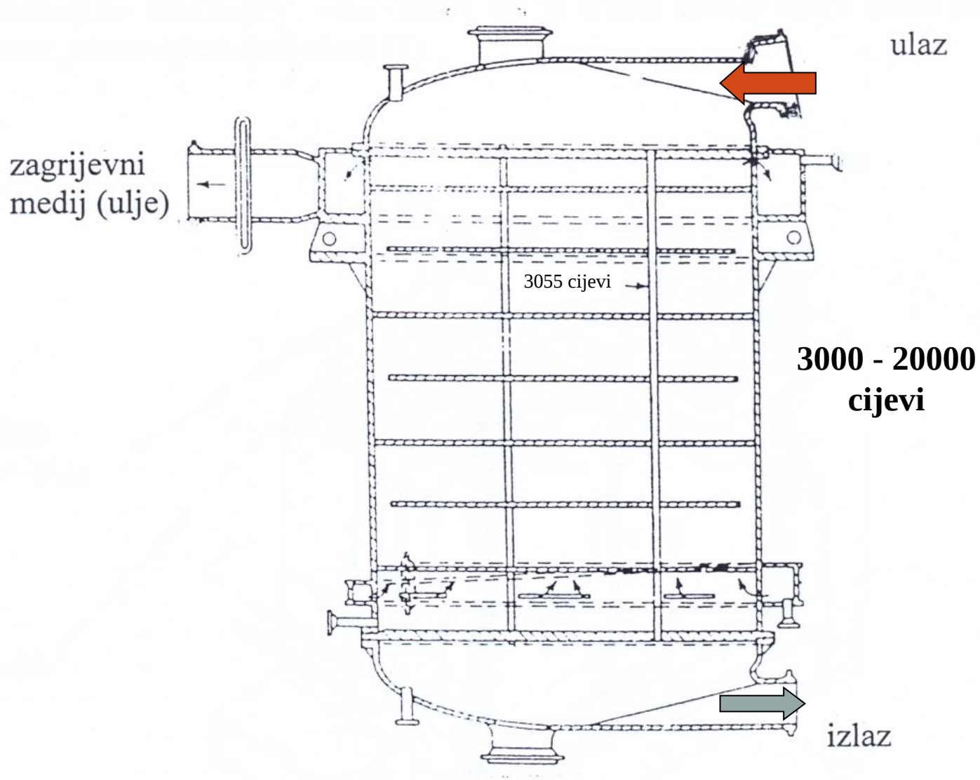
Reaktor izmjenjivač topline za sintezu ftalnog anhidrida.
