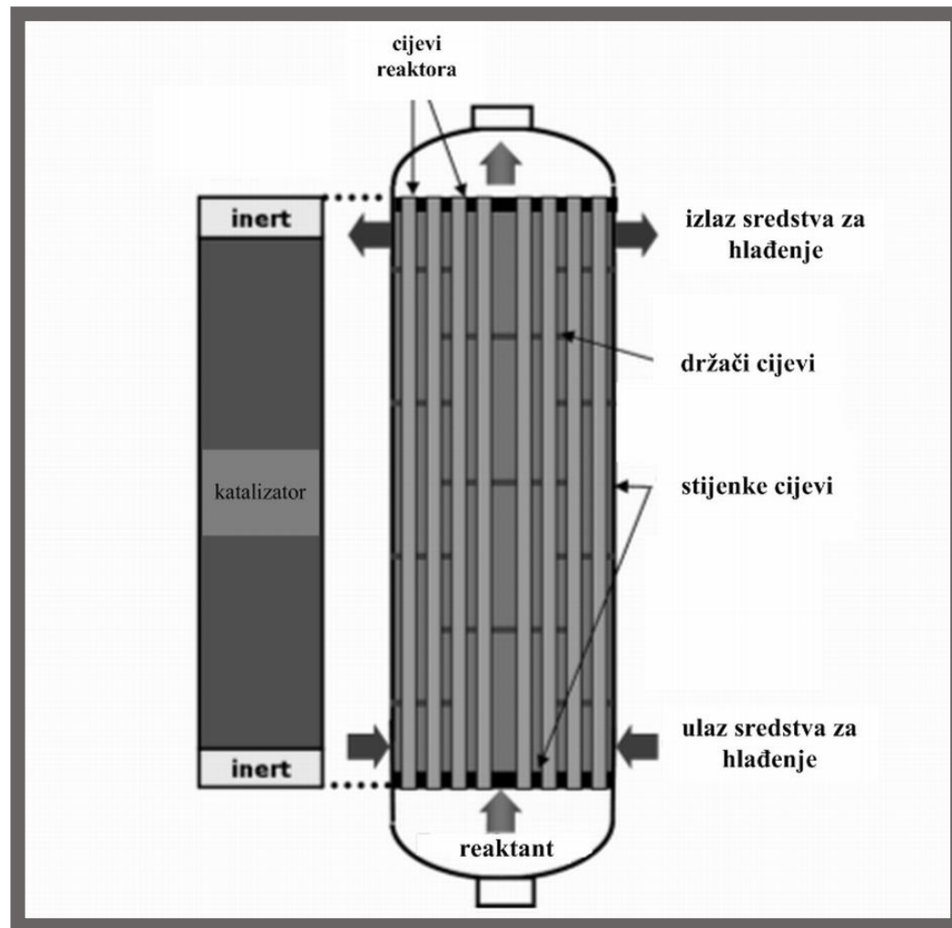
Reaktor- izmjenjivač topline
