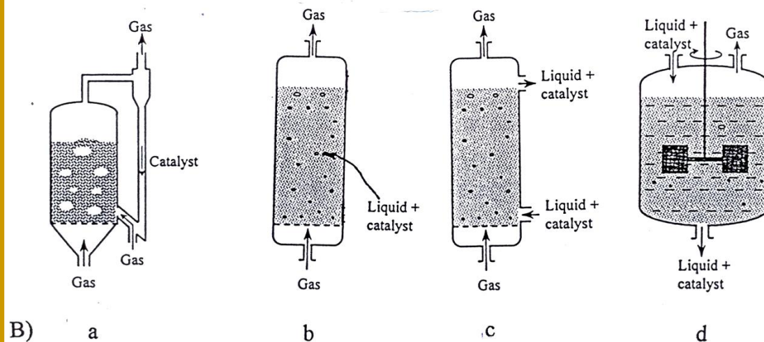
pokretni sloj katalizatora
