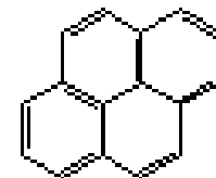
piren + CH 3
