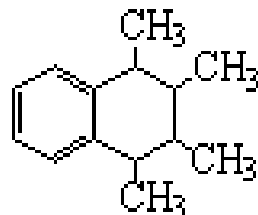
1,2,3,4-tetrametil tetralin
