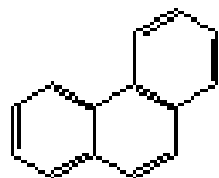
fenentren + CH 3
