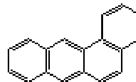
benzantracen
